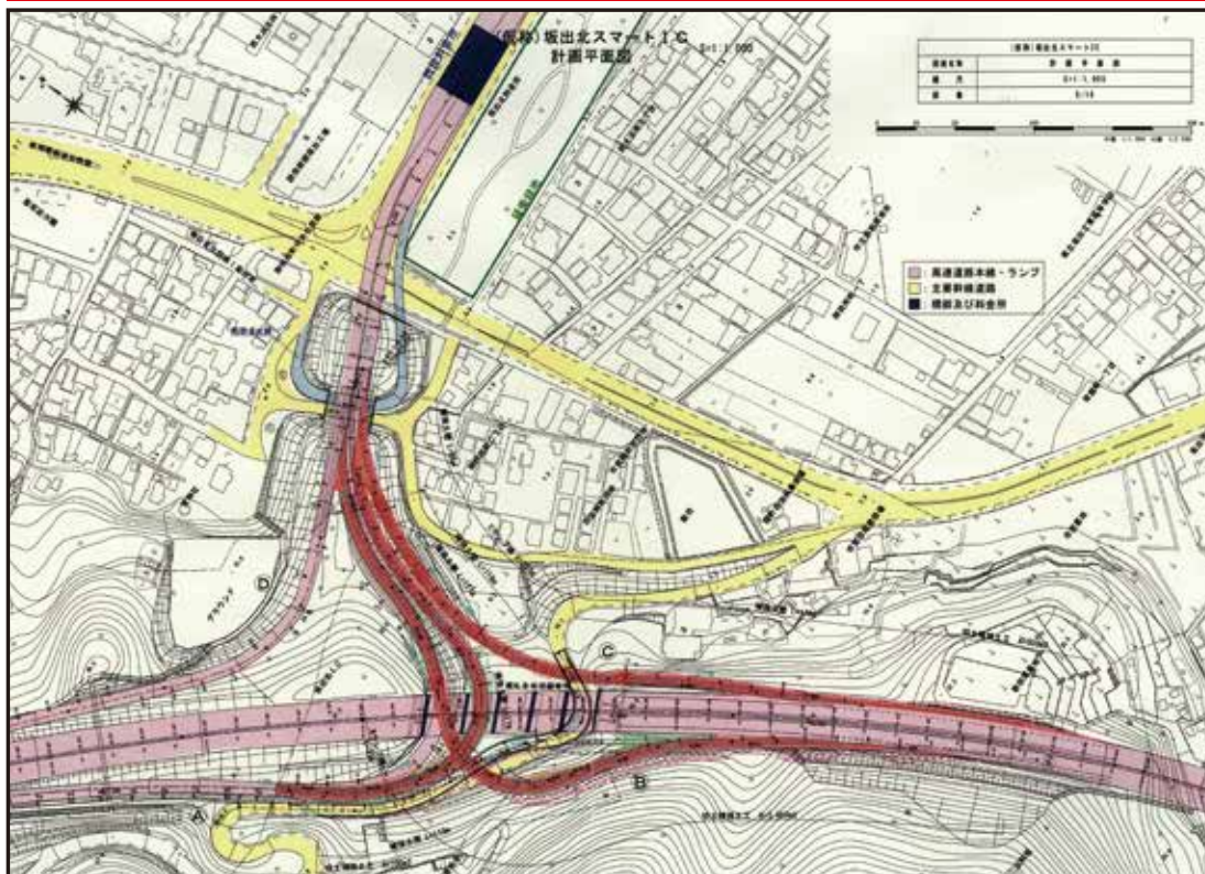
坂出北インターチェンジフル化 イメージ図
